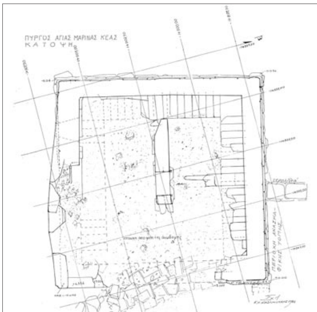
Σχέδιο 1. Κάτοψη του Πύργου της Αγίας Μαρίνας
