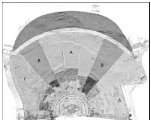
Κάτοψη του κοίλου στην οποία σημειώνονται οι τομείς που αντιστοιχούν στα στάδια του αναστηλωτικού προγράμματος (Σύνθεση επιμέρους αποτυπώσεων W. Wurster - Κ. Καζαμιάκη, Μ. Κορρέ και άλλων μελετητών Επιτροπής Διονυσιακού Θεάτρου - Α' ΕΠΚΑ).
