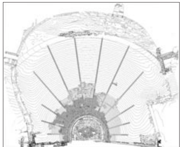
Κάτοψη της αναστηλωτικής πρότασης του κοίλου του Διονυσιακού Θεάτρου (Σχεδιαστικό υπόβαθρο: σύνθεση επιμέρους αποτυπώσεων W. Wurster - Κ. Καζαμάκη, Μ. Κορρέ και άλλων μελετητών Επιτροπής Διονυσιακού Θεάτρου - Α' ΕΠΚΑ).
