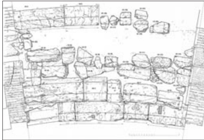
Κάτοψη της περιοχής του πιλοτικού προγράμματος αναστήλωσης στην κεντρική κερκίδα του μνημείου.
