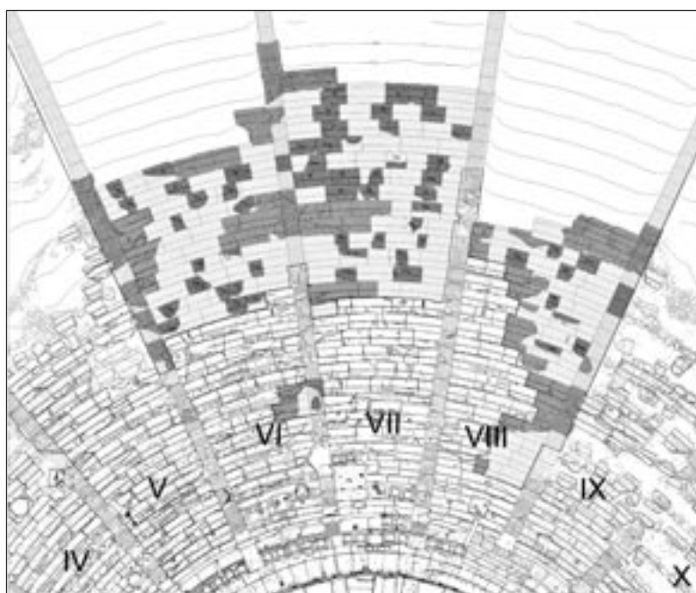
Πρόταση αναστήλωσης του κεντρικού τομέα (Α). Κάτοψη. Με ανοικτό τόνο σημειώνονται οι νέοι λίθοι, με ενδιάμεσο τόνο οι κατά χώραν σωζόμενοι και με σκούρο τόνο οι διάσπαρτοι επανεντασσόμενοι λίθοι (Σχεδιαστικό υπόβαθρο: αποτύπωση W. Wurster - Κ. Καζαμάκη).
