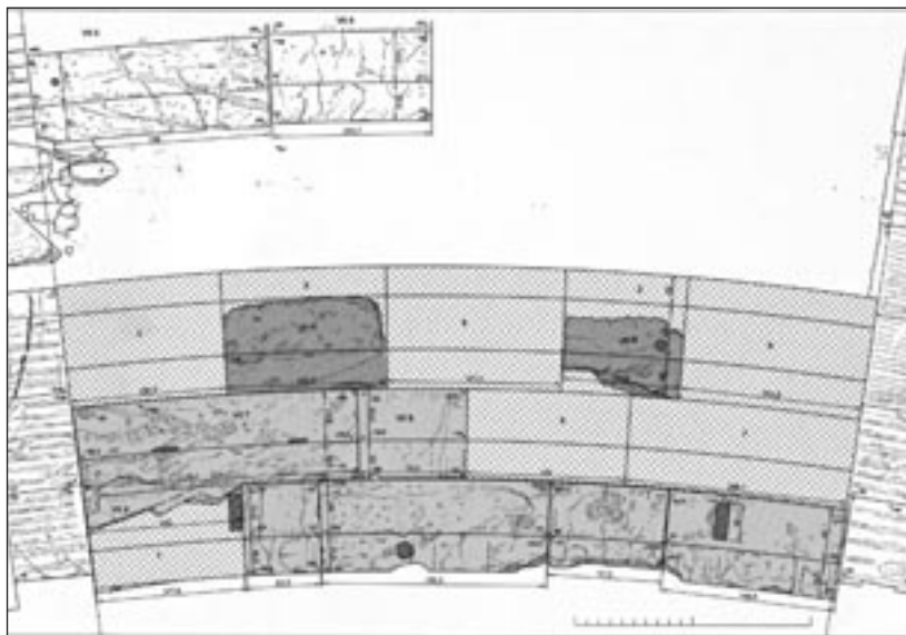
Κάτοψη της αναστηλωτικής πρότασης για την περιοχή του πιλοτικού προγράμματος.
