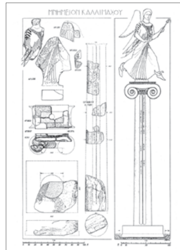
Το μνημείο του Καλλιμάχου: Γραφική αποκατάσταση του Μ. Κορρέ
